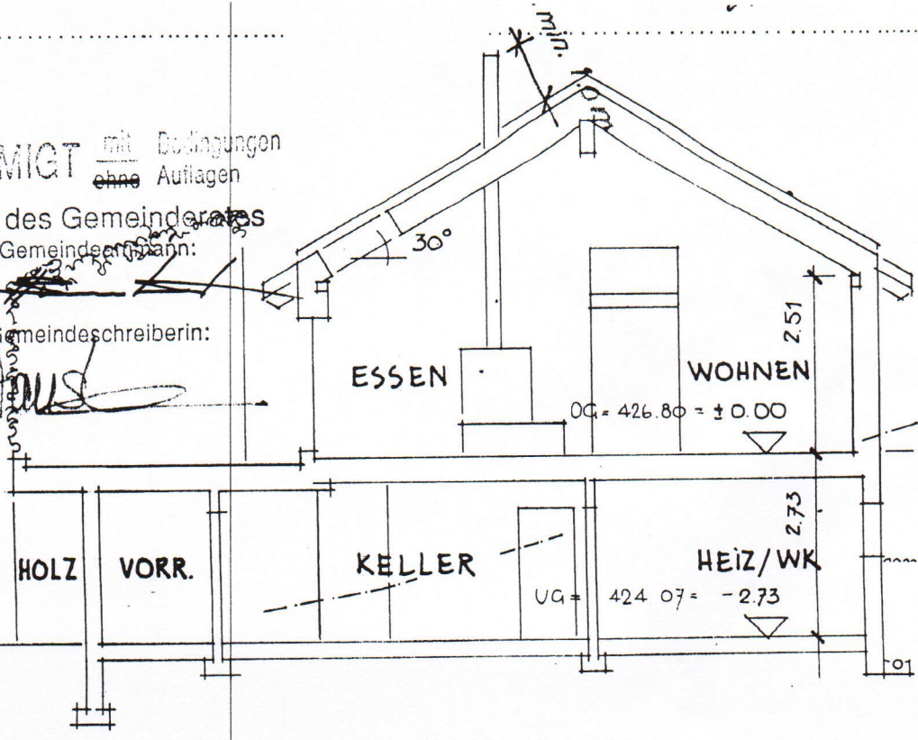
SCHNITT 1--1
