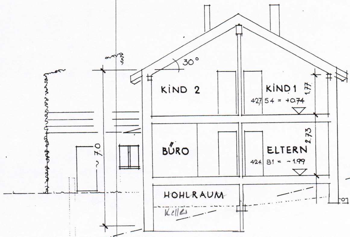
SCHNITT 2--2
